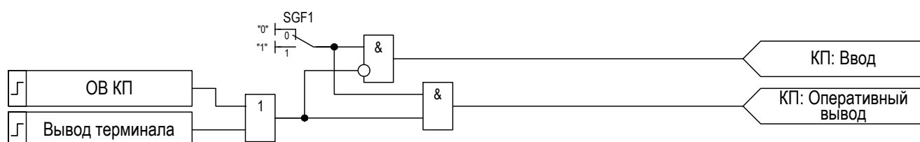
Рисунок 2.54 – Функциональная схема управления режимами работы функционального блока «КП»
