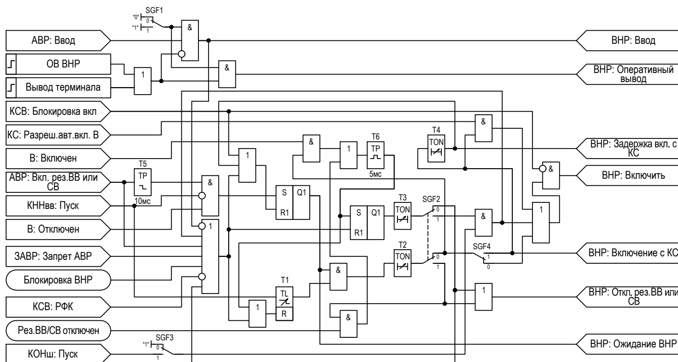
Рисунок 2.47 – Функциональная схема «ВНР»
