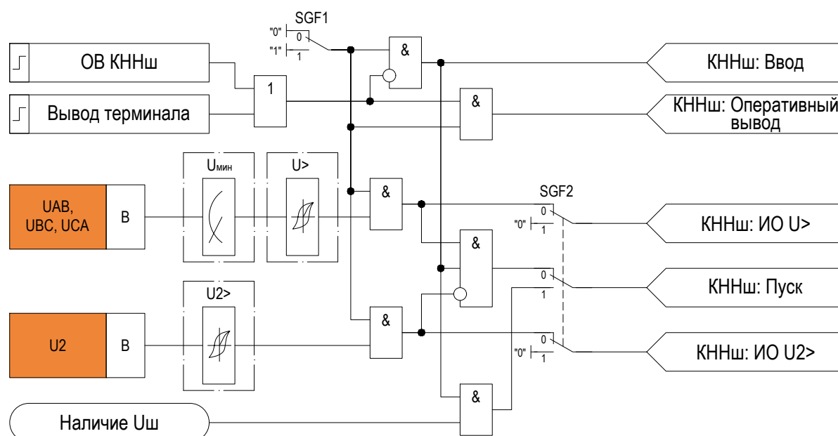
Рисунок 2.41 – Функциональная схема «КННш»
