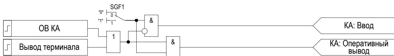
Рисунок 2.70 – Логика управления режимами функционального блока «КА»
