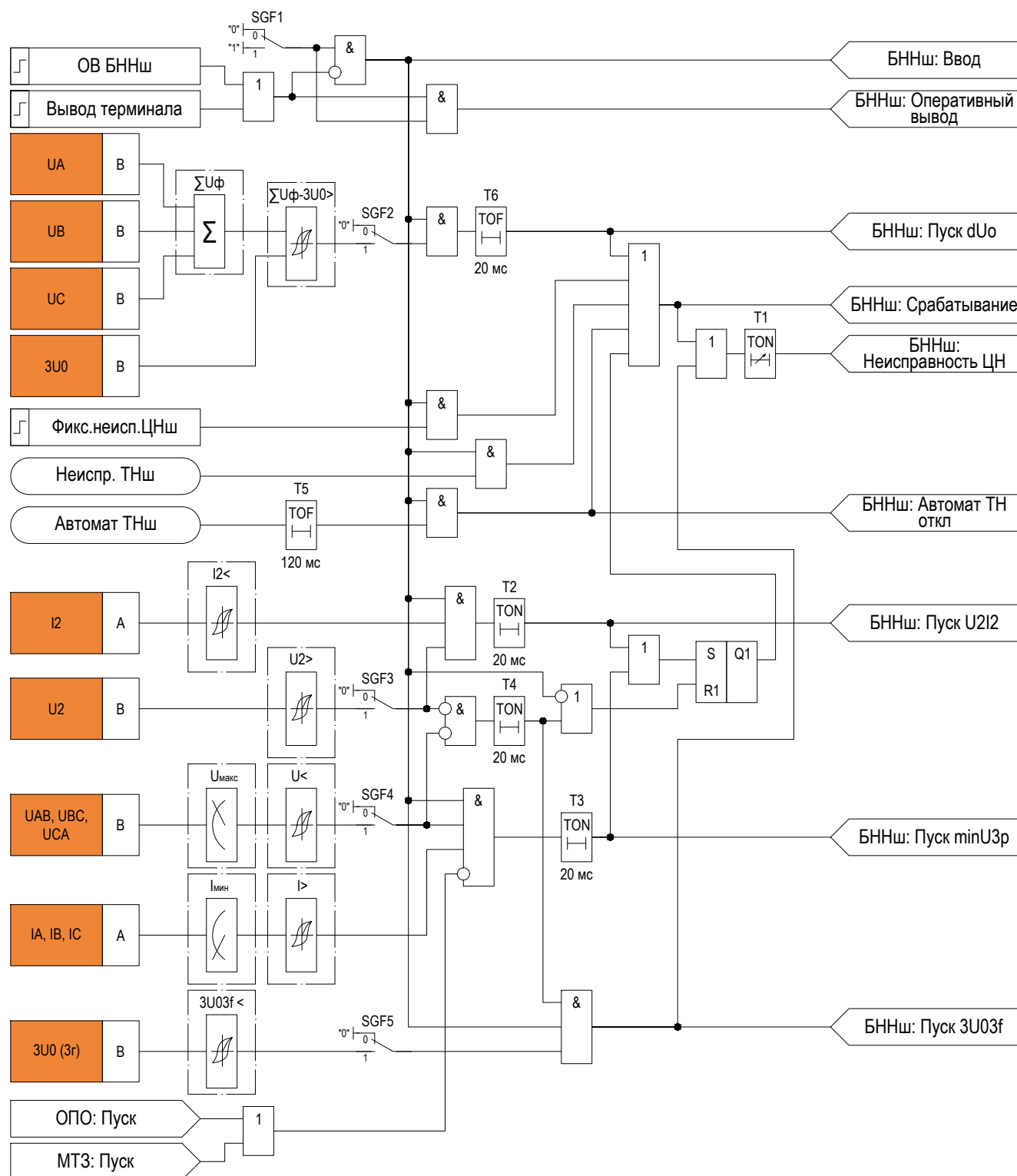
Рисунок 2.38 – Функциональная схема «БННш»
