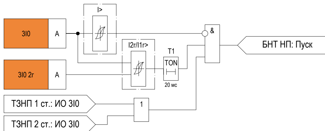
Рисунок 2.33 – Функциональная схема «БНТ НП»
