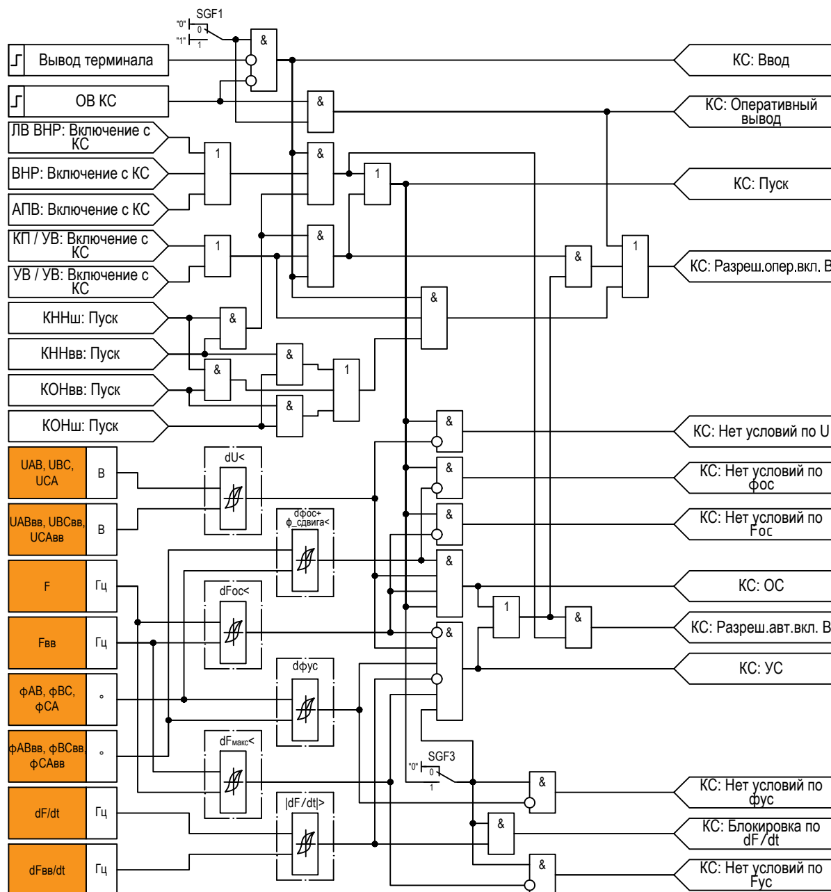
Рисунок 2.48 – Функциональная схема «КС»
