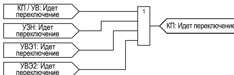
Рисунок 2.55 – Функциональная схема формирования общего сигнала переключения коммутационного аппарата
