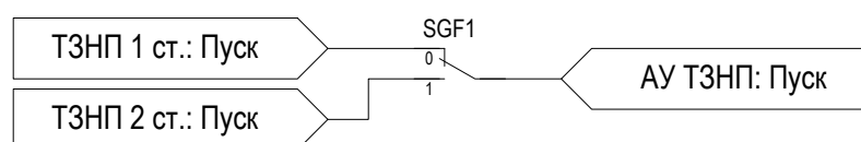
Рисунок 2.34 – Функциональная схема АУ ТЗНП
