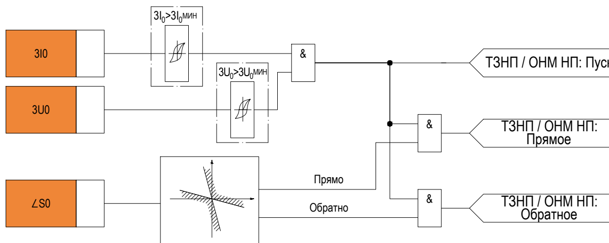
Рисунок 2.32 – Функциональная схема «ОНМ НП»
