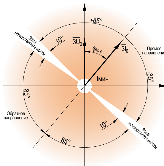
Рисунок 2.31 – Характеристика органа направления мощности нулевой последовательности
