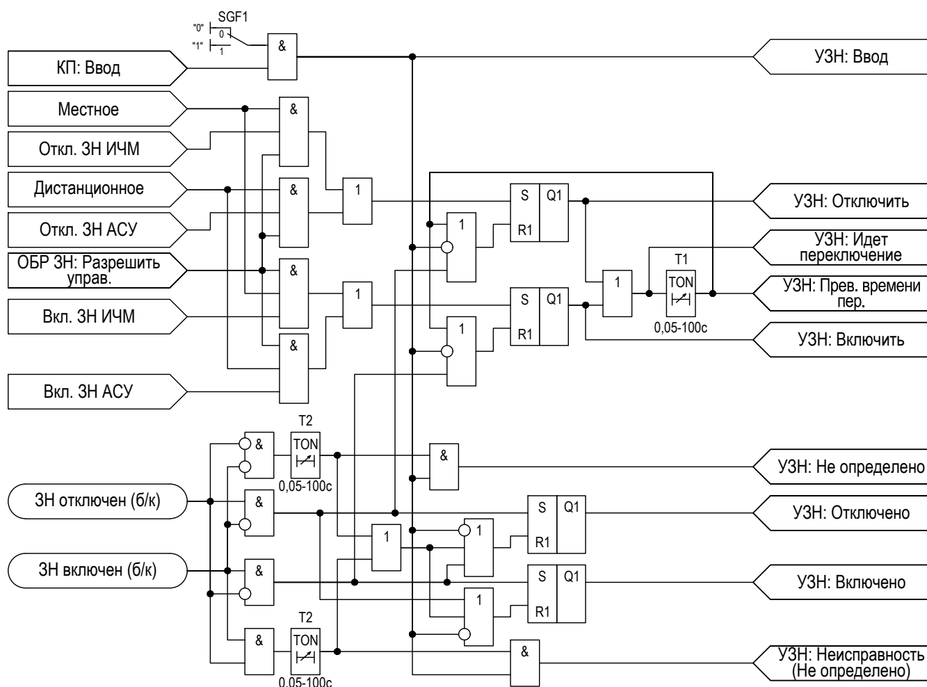
Рисунок 2.57 – Функциональная схема «УЗН»
