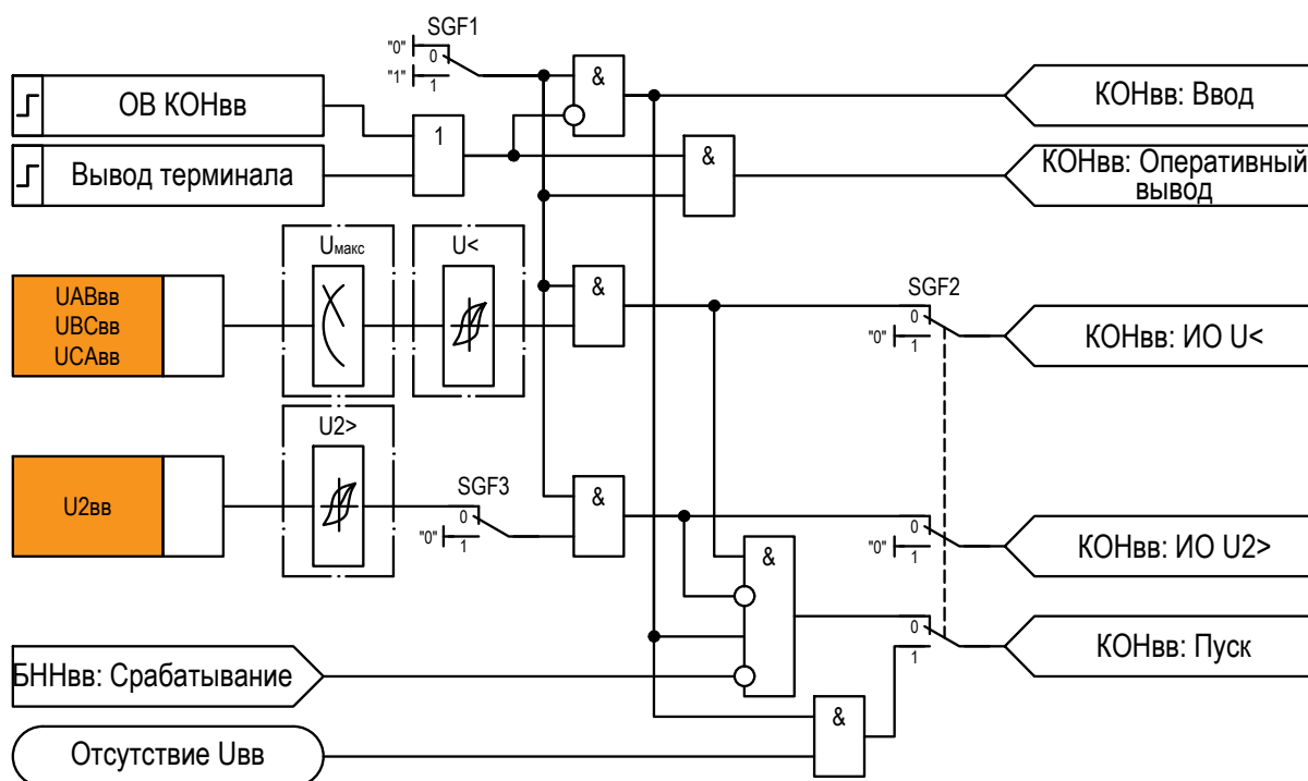
Рисунок 2.44 – Функциональная схема «КОНвв»
