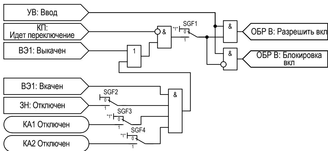
Рисунок 2.60 – Функциональная схема «ОБР В»
