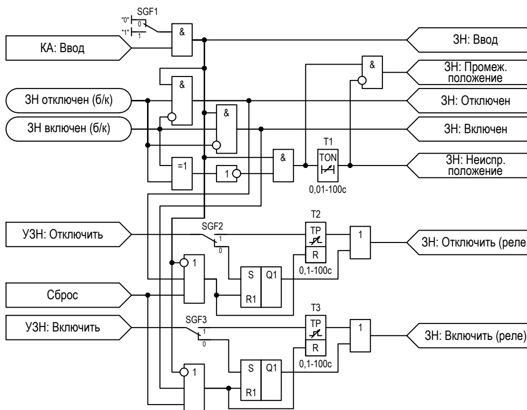
Рисунок 2.73 – Функциональная схема «ЗН»
