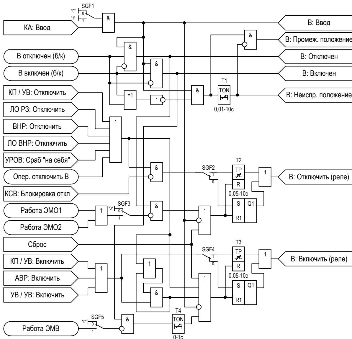
Рисунок 2.72 – Функциональная схема «Выключатель»
