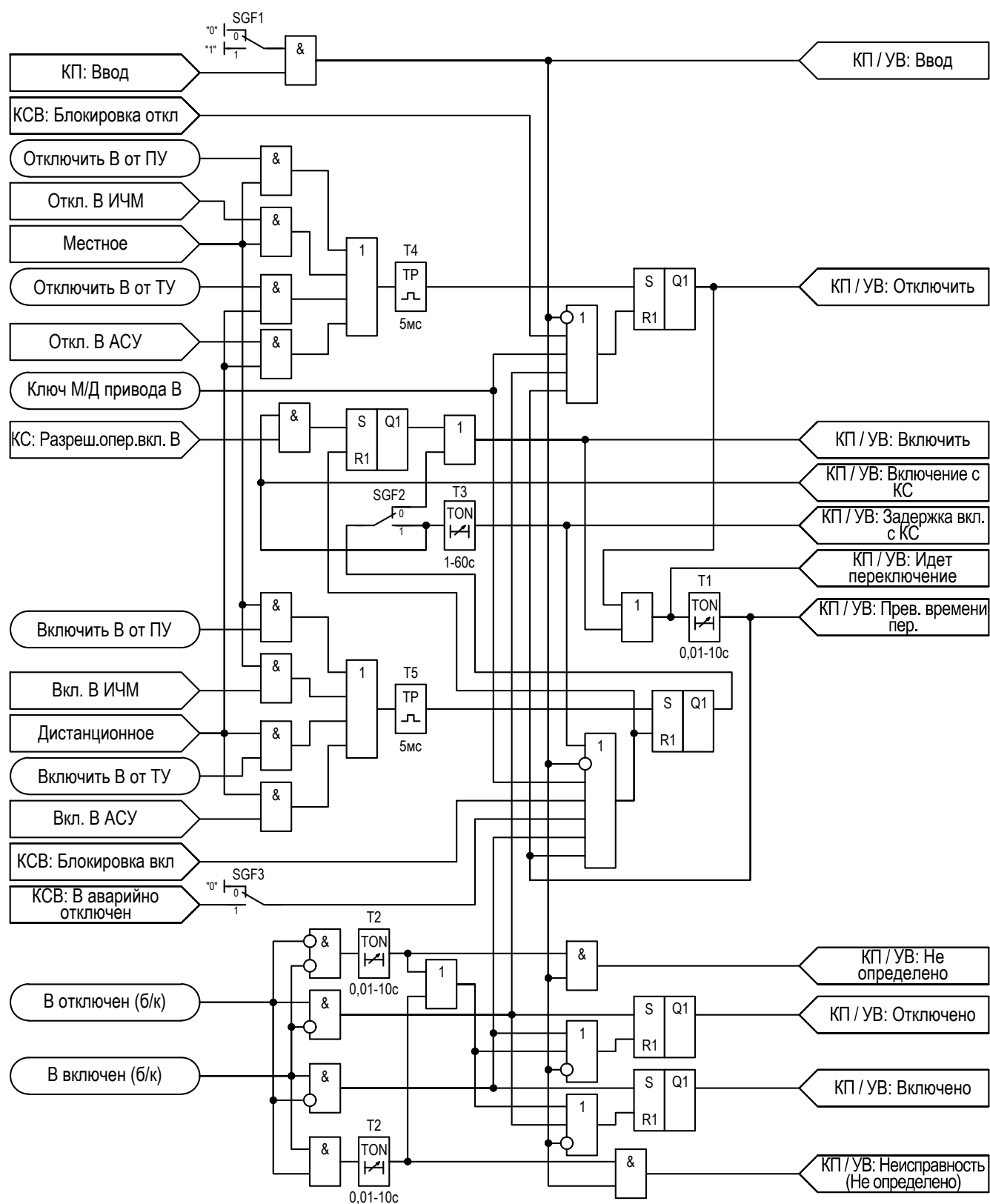
Рисунок 2.56 – Функциональная схема «УВ»
