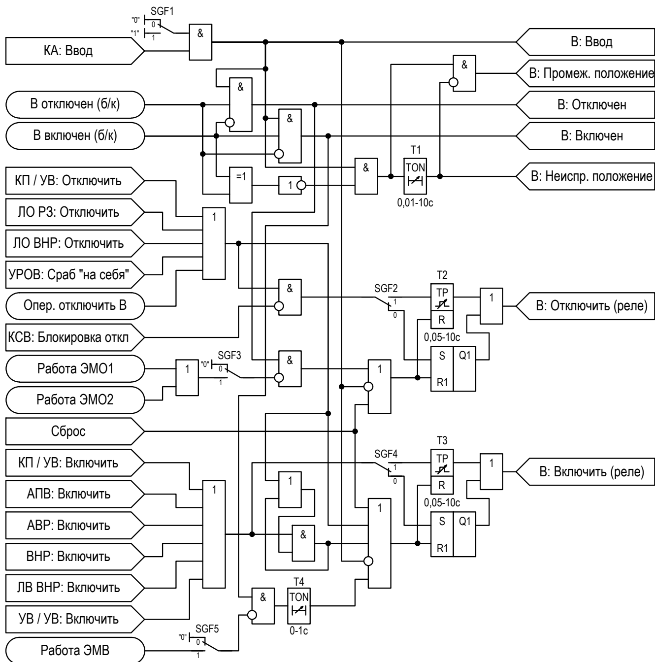
Рисунок 2.71 – Функциональная схема «Выключатель»
