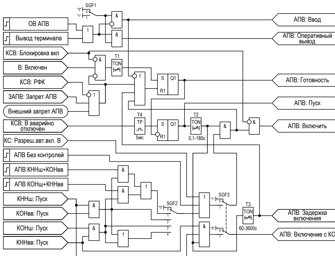
Рисунок 2.40 – Функциональная схема «АПВ»
