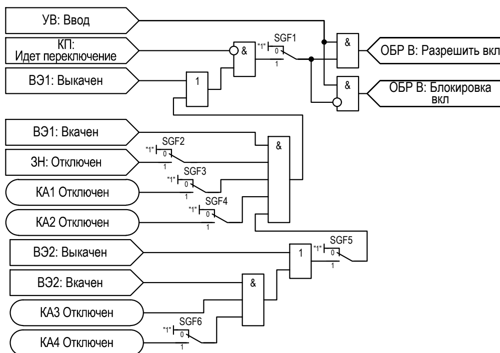
Рисунок 2.65 – Функциональная схема «ОБР В»
