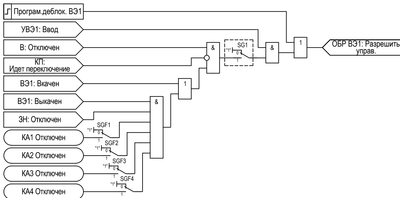
Рисунок 2.62 – Функциональная схема «ОБР ВЭ1»
