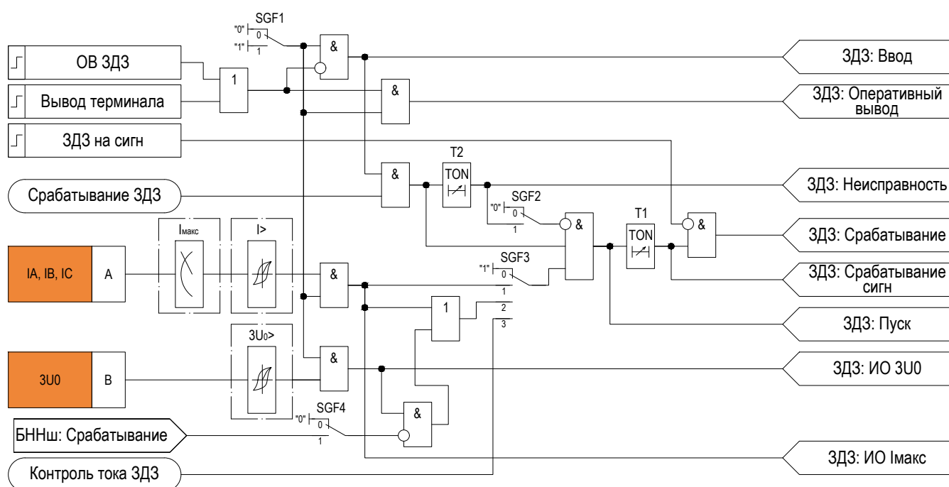
Рисунок 2.26 – Функциональная схема «ЗДЗ»
