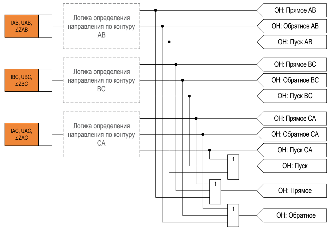
Рисунок 2.8 – Функциональная схема «ОН»
