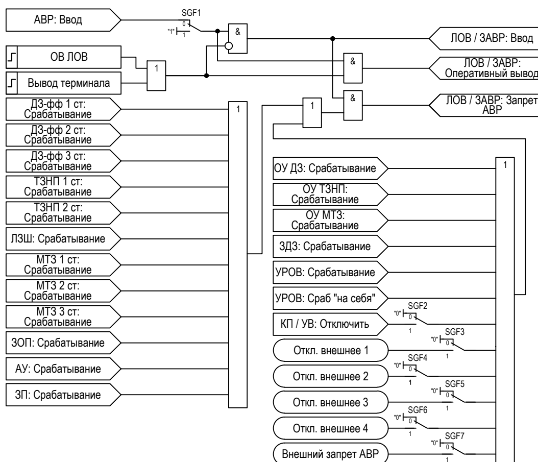
Рисунок 2.53 – Функциональная схема «ЗАВР ЛО»
