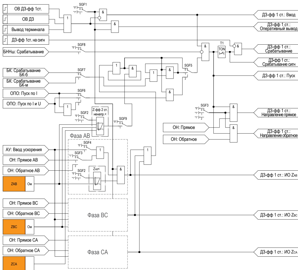
Рисунок 2.3 – Функциональная схема «ДЗ-фф 1ст.»
