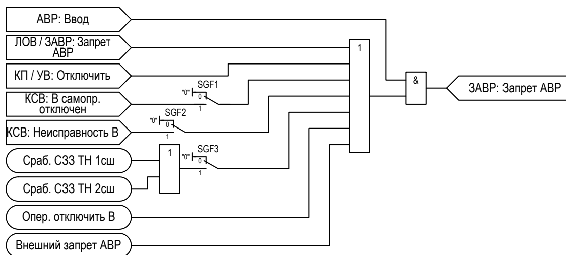
Рисунок 2.46 – Функциональная схема «ЗАВР»
