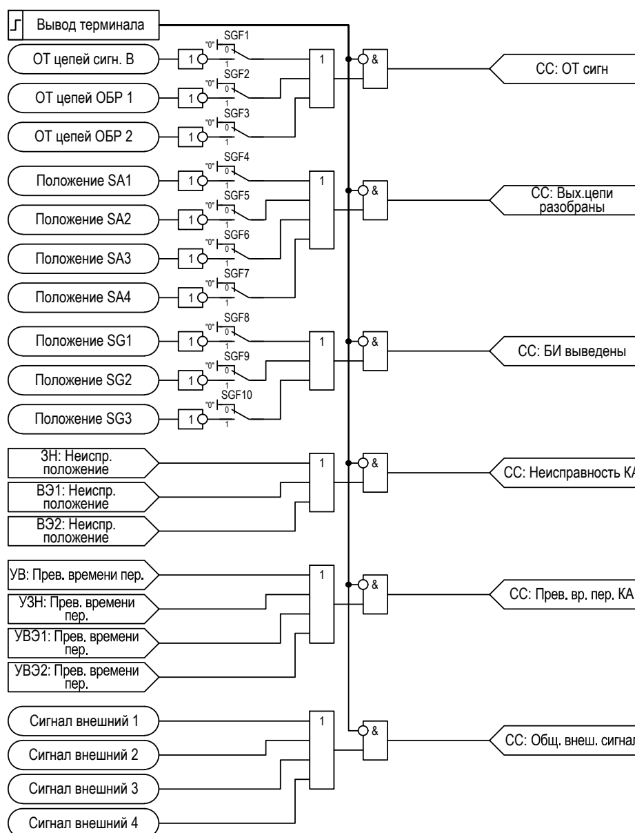
Рисунок 2.77 – Функциональная схема «СС»
