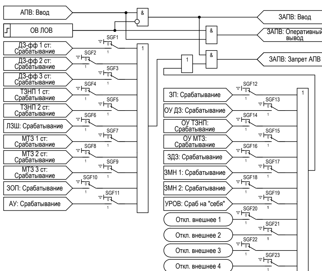
Рисунок 2.52 – Функциональная схема «ЗАПВ»
