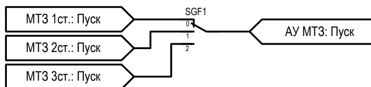
Рисунок 2.23 – Функциональная схема АУ МТЗ
